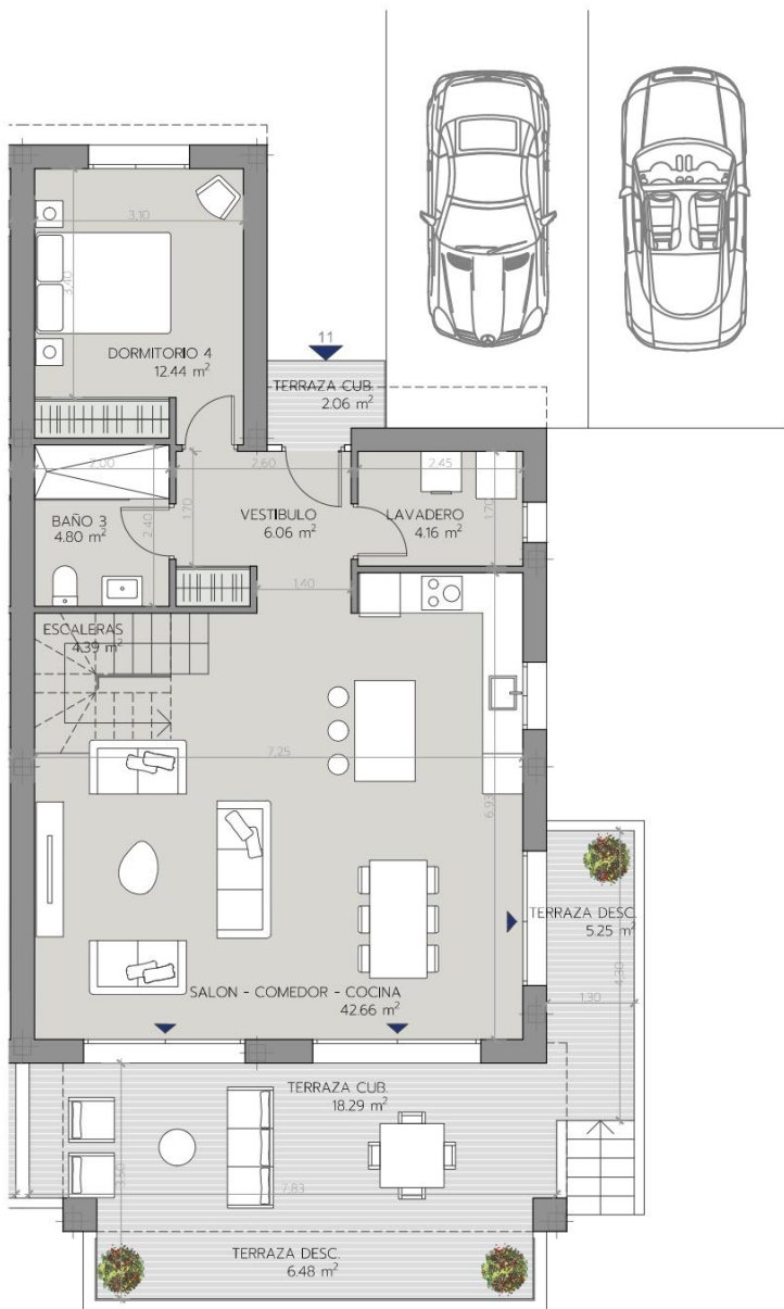
PLANTA BAJA
