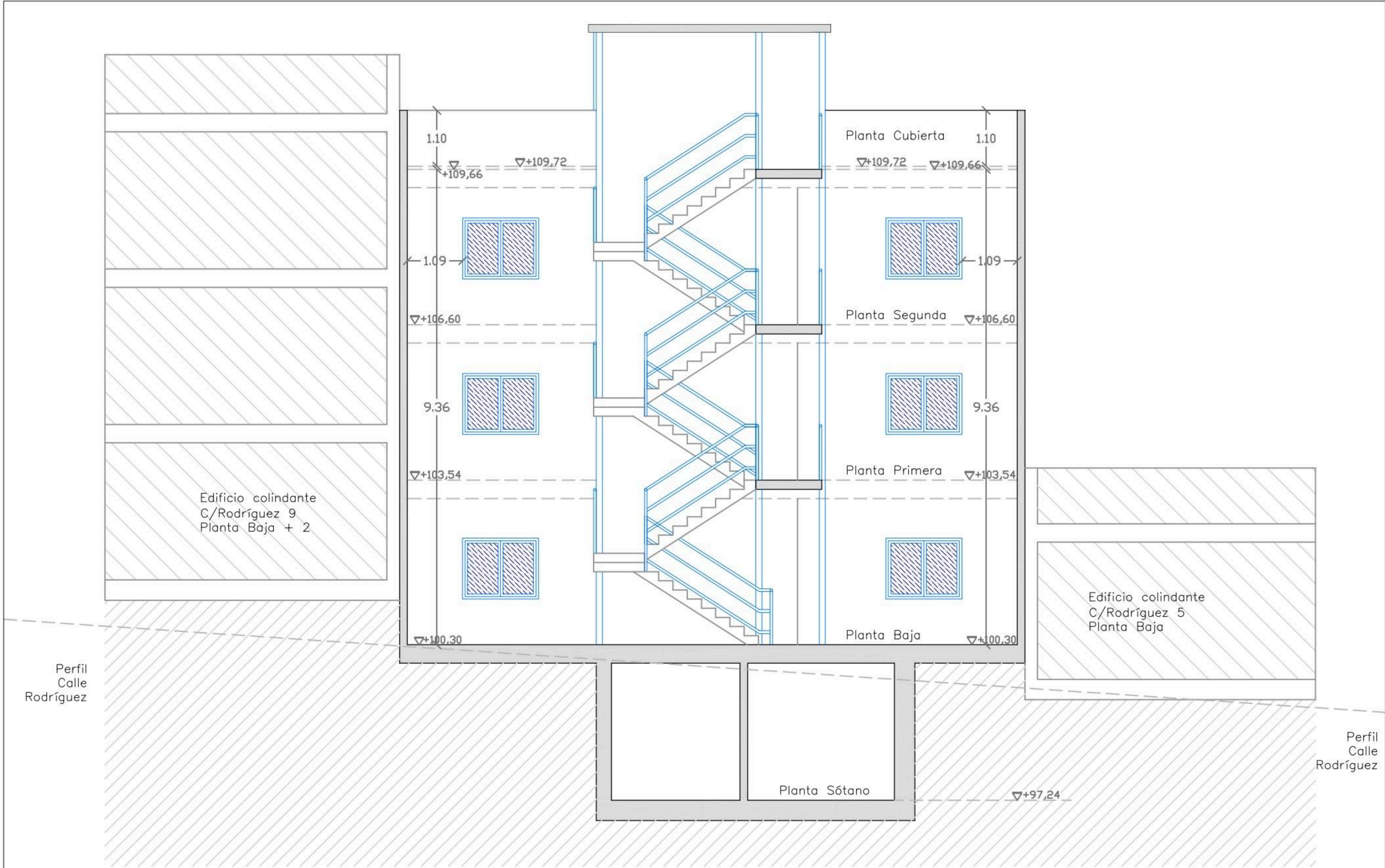
ALZADO INTERIOR BLOQUE A
