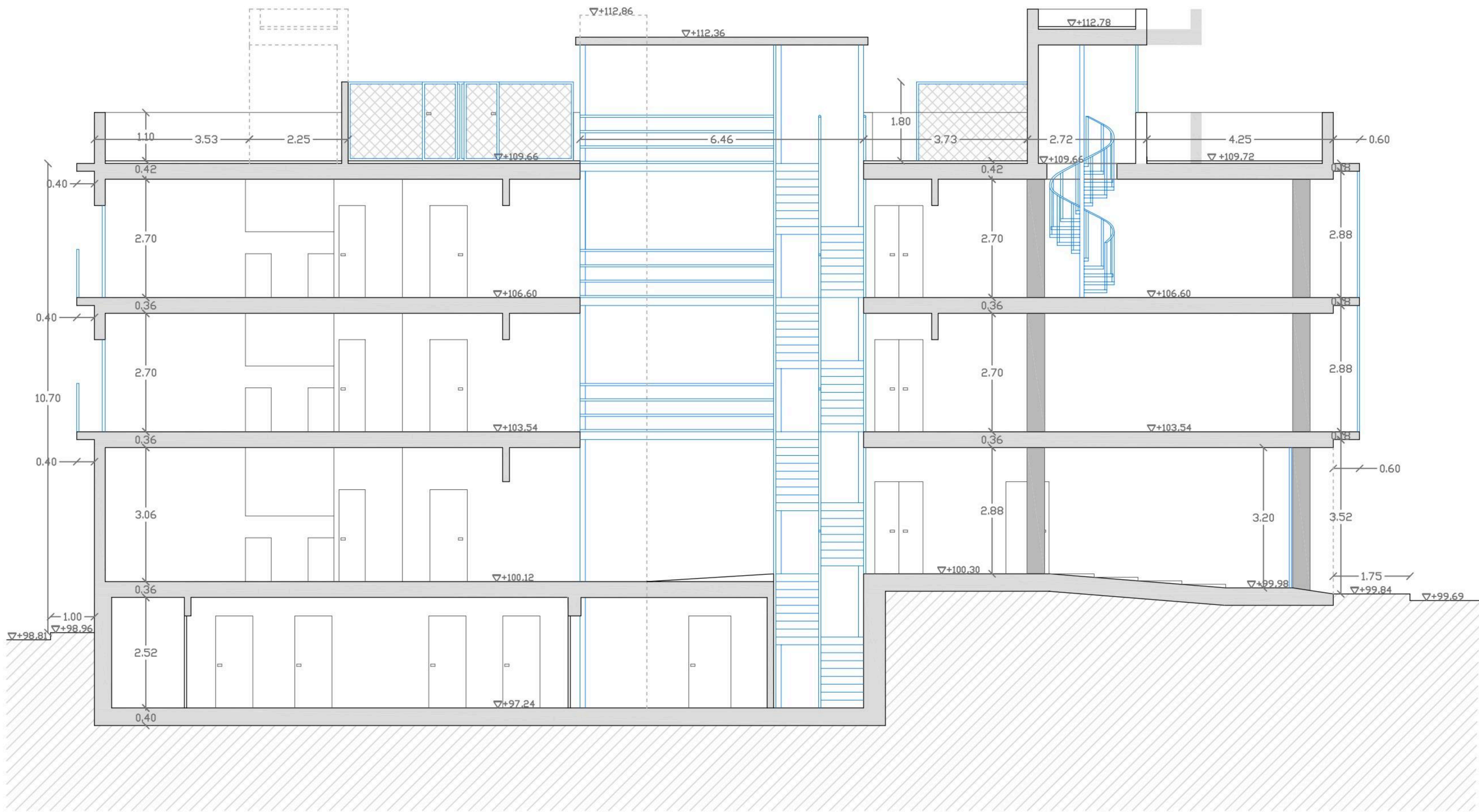
SECCIÓN A-A'
