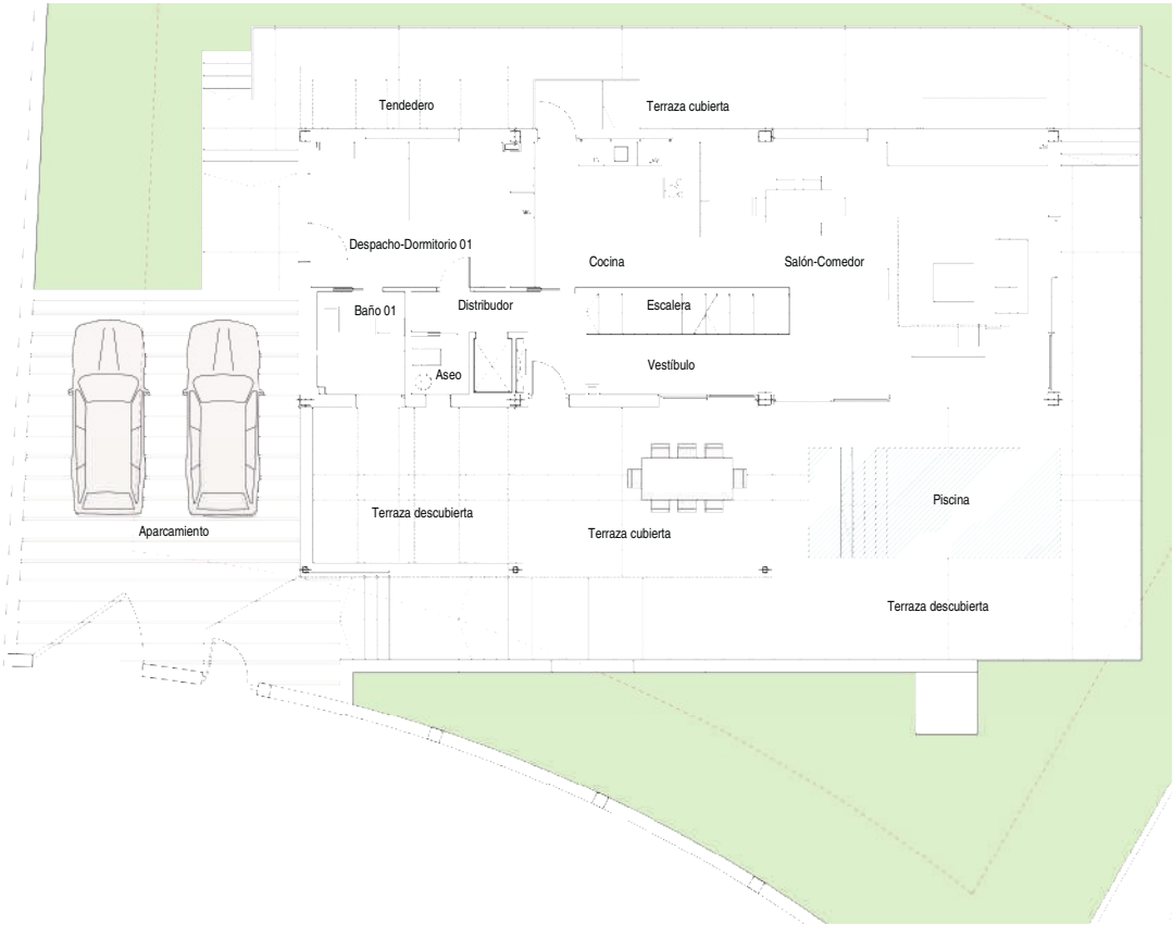
Planta Baja
